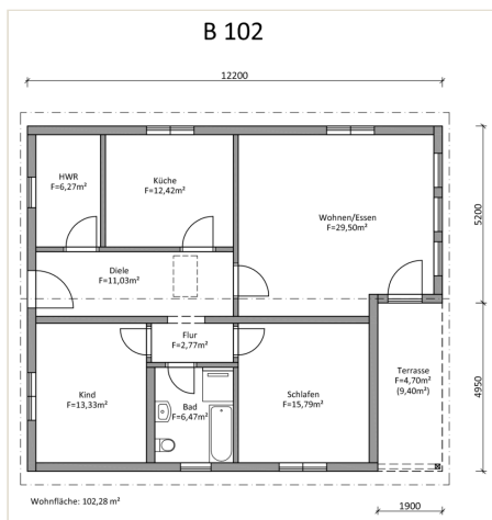
Erdgeschoss
