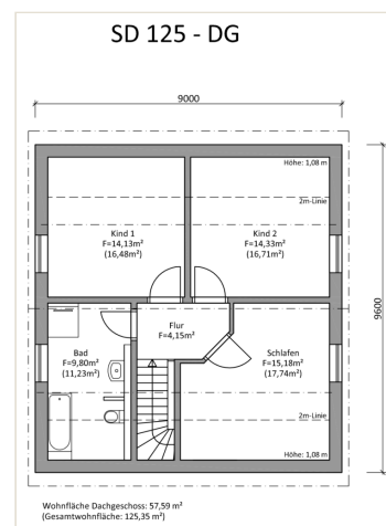
Obergeschoss
