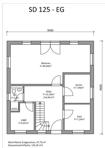
Erdgeschoss
