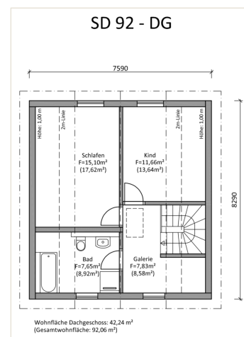
Obergeschoss
