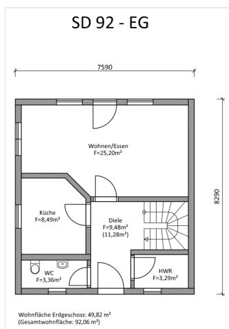
Erdgeschoss
