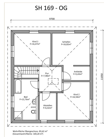
Obergeschoss
