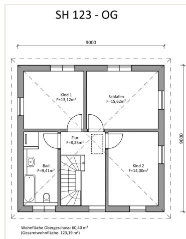
Obergeschoss
