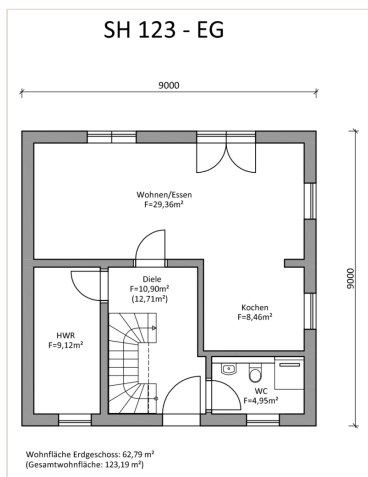
Erdgeschoss
