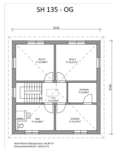
Obergeschoss
