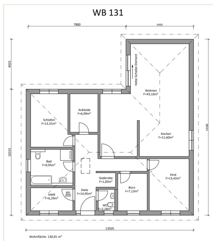
Erdgeschoss
