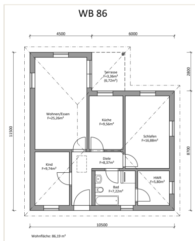
Erdgeschoss
