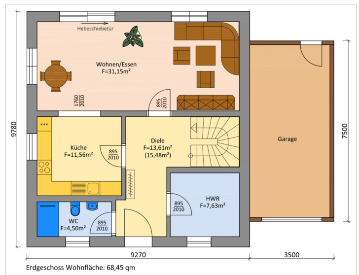
Erdgeschoss
